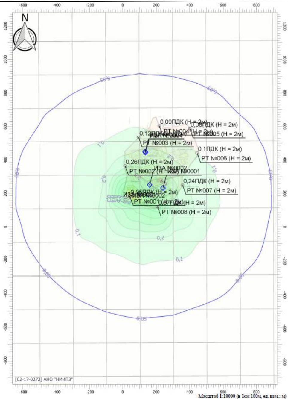
Рисунок 4.4.1.10 – Зона влияния выбрасываемых веществ на уровне 0,05 ПДК (шаг сетки 200 м)
