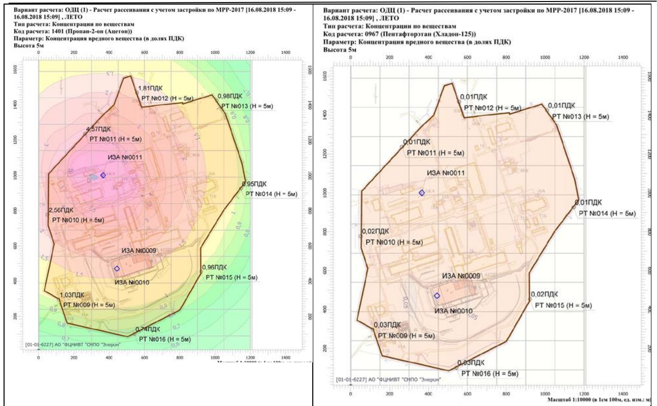
Рисунок 4.5.1.1 – Результат расчета рассеивания выброса ЗВ при аварийной ситуации
