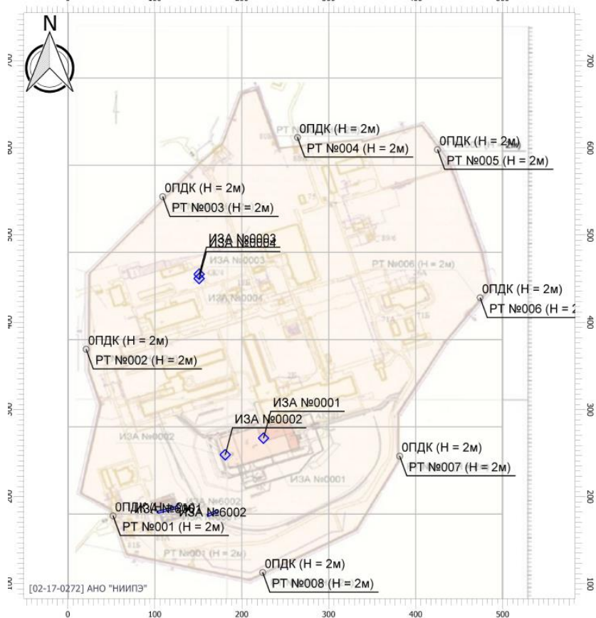
Рисунок 4.4.1.9 – Расчет рассеивания 2752 Уайт-спирит
