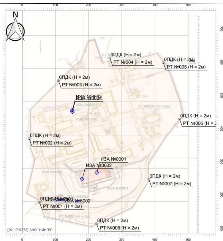
Рисунок 4.4.1.4 – Расчет рассеивания 0621 Метилбензол (Толуол)
