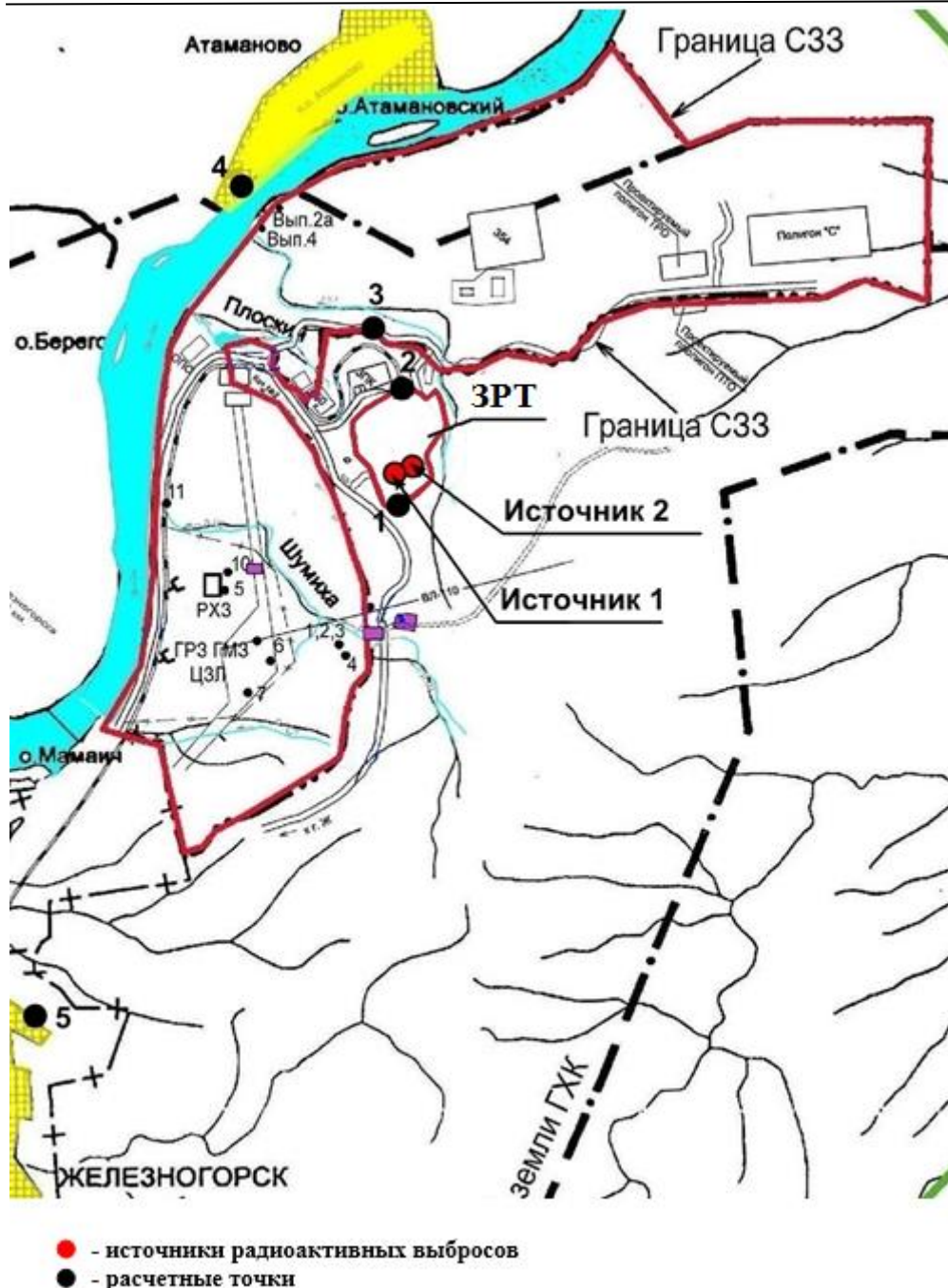
Рисунок 4.4.4.1 - Ситуационный план-схема размещения ОДЦ с указанием источников радиоактивных выбросов и расчетных точек
