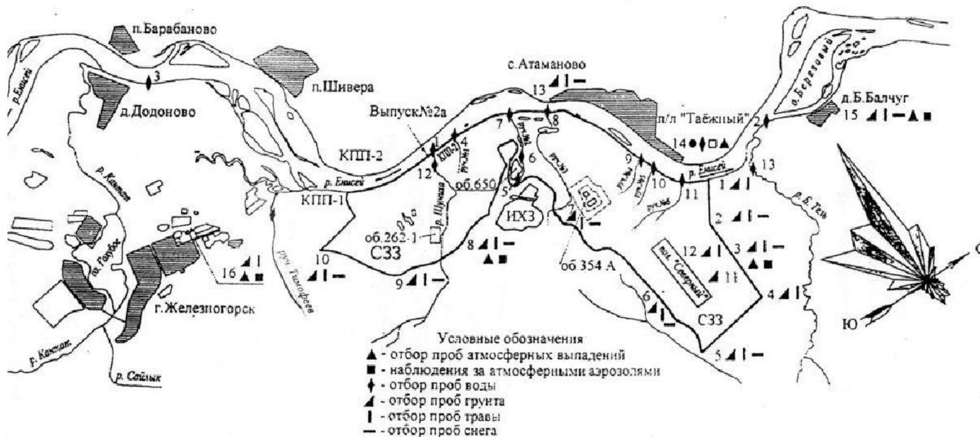
Рис. 4.8.1 Карта-схема расположения пунктов радиометрического контроля
