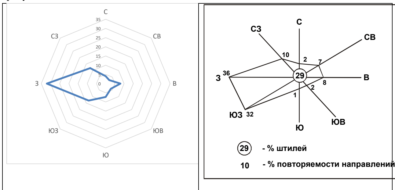
Рисунок 4.3.2.1 - Роза ветров по мс Шалинское и г. Красноярск
